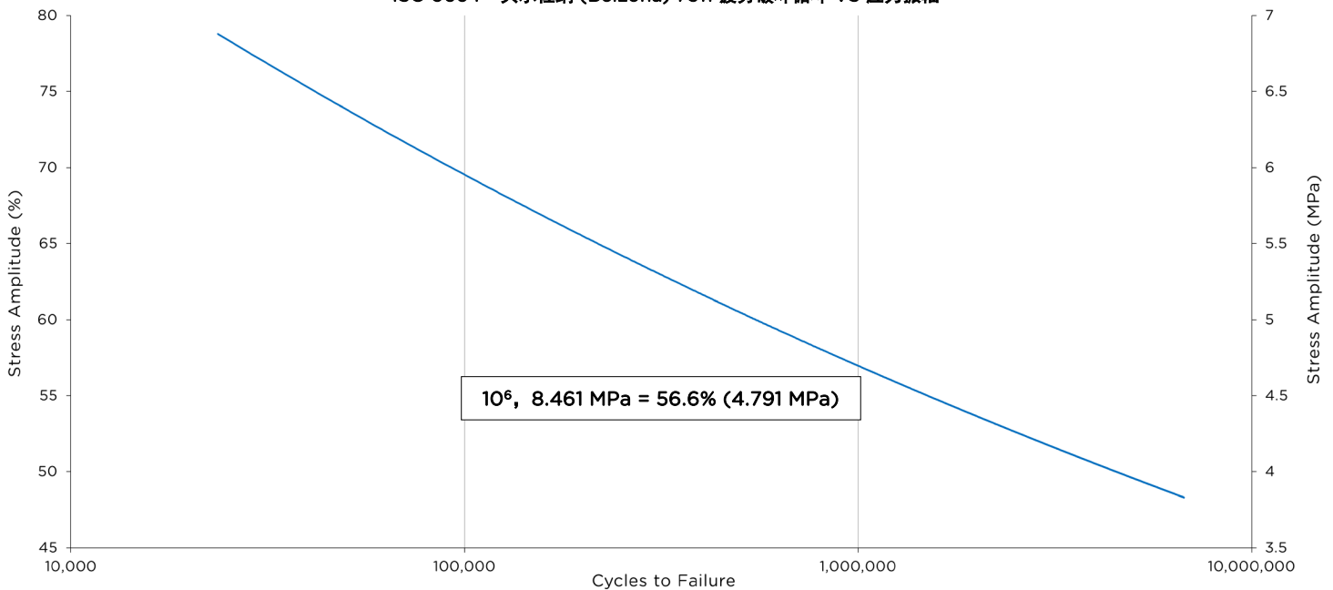
ISO 9664 - 贝尔佐纳 (Belzona) 7311 疲劳破坏循环 VS 应力振幅
